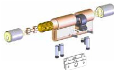
Zvýšená odolnost proti vytržení díky ocelovým lamelám a kaleným stavítkům a šroubům pro upevnění insertu
